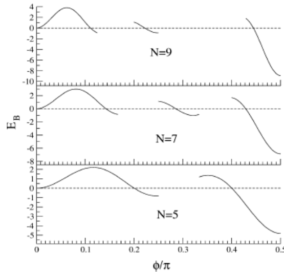
شکل ۲: انرژی پیوند حالت سالتون N -ذره‌ای بر حسب \phi/\pi برای سه مقدار مختلف N [۴].
